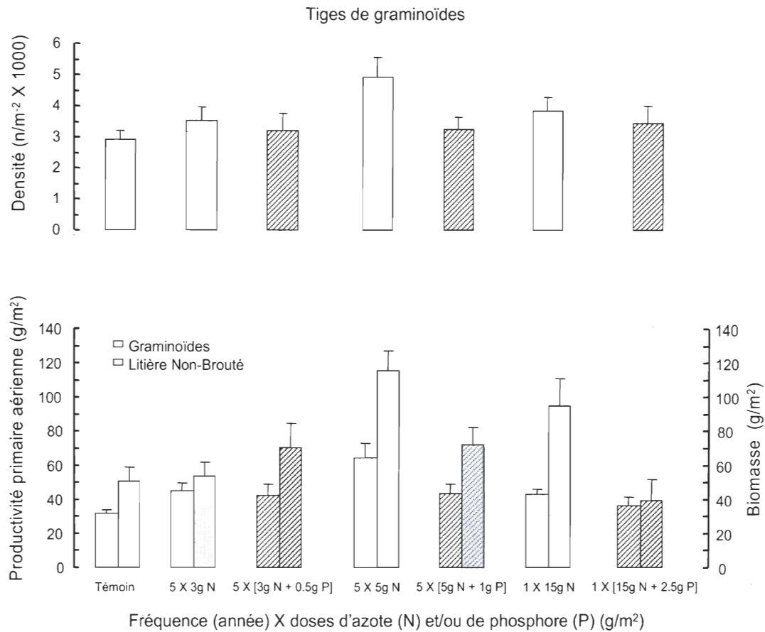
Figure 3.7: Productivité primaire aérienne ( g/m^2 ) et densité en tiges ( n/m^2 ) des graminoides et biomasse de la litière du traitement Non-broué en fonction du type de fertilisation en azote (seul \square ou en combinaison avec le phosphore \square ), après cinq saisons de croissance dans les polygones de tourbe de l'île Bylot. Les barres hachurées mettent l'emphase sur les traitements combinés (N+P). Moyenne \pm erreur-type, graminoides et tiges ( n=12 /traitement), litière Non-broué ( n=6 /traitement). Voir tableau 3.1 et 3.2 pour les valeurs de ( p ).
