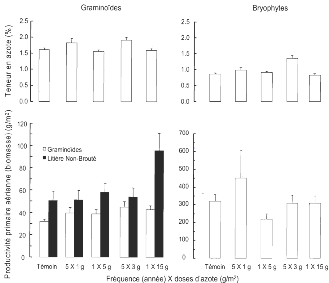
Figure 3.5: Productivité primaire aérienne ( \text{g/m}^2 ) et teneur en azote total (%) des graminoides et des bryophytes et biomasse de la litière du traitement Non-broué, en fonction de la fréquence d'application des fertilisants azotés inorganiques (individuelle ou annuelle), après cinq saisons de croissance dans les polygones de tourbe de l'île Bylot. Moyenne \pm erreur-type, graminoides et bryophytes ( n=12/\text{traitement} ), litière Non-broué ( n=6/\text{traitement} ). Voir tableau 3.1 et 3.2 pour les valeurs de ( p ).
