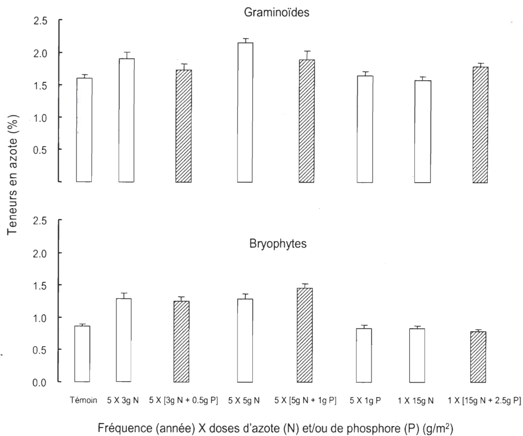
Figure 3.8: Teneurs en azote total (%) des graminoides et des bryophytes en fonction du type de fertilisation azotée ou phosphorée (seule □ ou en combinaison avec le phosphore ou l'azote ▨), après cinq saisons de croissance dans les polygones de tourbe de l'île Bylot. Les barres hachurées mettent l'emphase sur les traitements combinés (N+P). Moyenne \pm erreur-type, (n=12/traitement). Voir tableau 3.2 pour les valeurs de ( p ).
