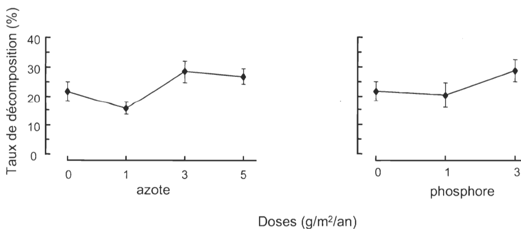
Figure 3.10: Taux de décomposition (%) de la matière organique du traitement Non-brouté, en fonction des traitements d'azote et de phosphore inorganiques annuels ( \text{g/m}^2/\text{an} ), après cinq saisons de croissance dans les polygones de tourbe de l'île Bylot. Moyenne \pm erreur-type, ( n=6/\text{traitement} ). Voir tableau 3.4 pour les valeurs de ( p ).
