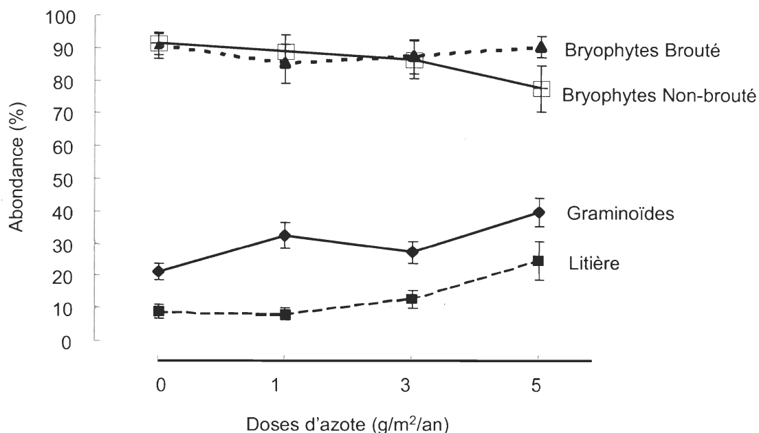
Figure 3.2: Abondance (%) des plantes graminoides ( Eriophorum , Dupontia , Carex ), de la litière et des bryophytes en fonction des traitements d'azote inorganique annuels ( \text{g/m}^2/\text{an} ), après cinq saisons de croissance dans les polygones de tourbe de l'île Bylot. Moyenne \pm erreur-type, graminoides et litière ( n=48 ), bryophytes Brouté et Non-brouté ( n=24 ). Voir tableau 3.3 pour les valeurs de ( p ).
