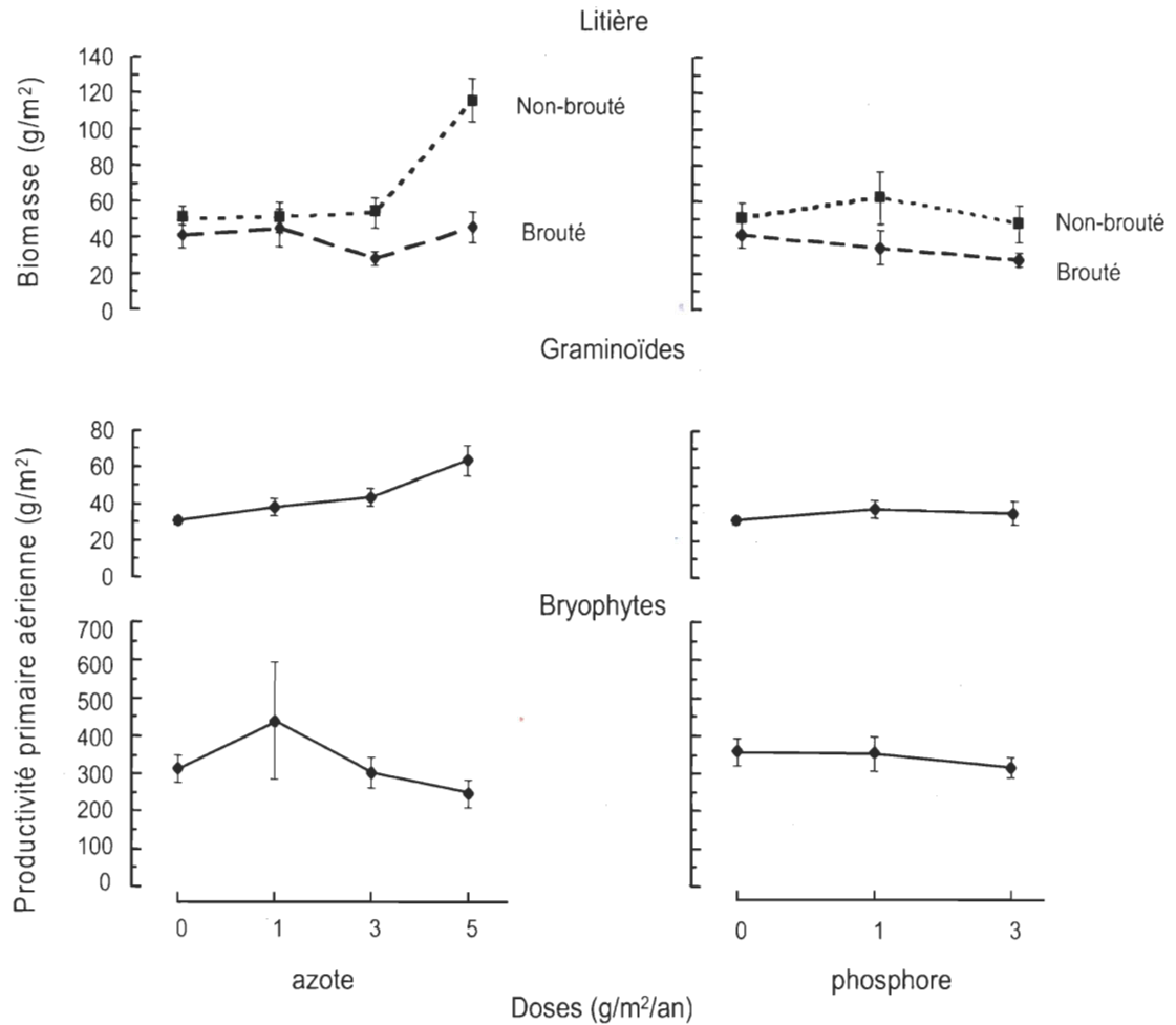
Figure 3.3: Productivité primaire (g/m 2 ) des bryophytes, des plantes graminoides ( Eriophorum , Dupontia , Carex ) et biomasse de la litière (g/m 2 ) en fonction des traitements d'azote et de phosphore inorganiques annuels (g/m 2 /an), après cinq saisons de croissance dans les polygones de tourbe de l'île Bylot. Moyenne \pm erreur-type, graminoides et bryophytes (n=12/traitement), litière Brouté ou Non-brouté (n=6/traitement). Voir tableau 3.1 pour les valeurs de ( p ).
